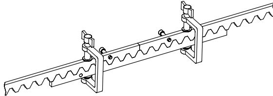
Рисунок 8. Позиционирование реек
