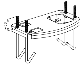
Малюнок 3. Монтажна основа
